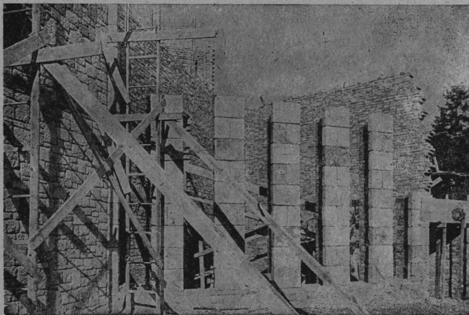
Épül az Utolsó Vacsora termének lépcsőháza.
