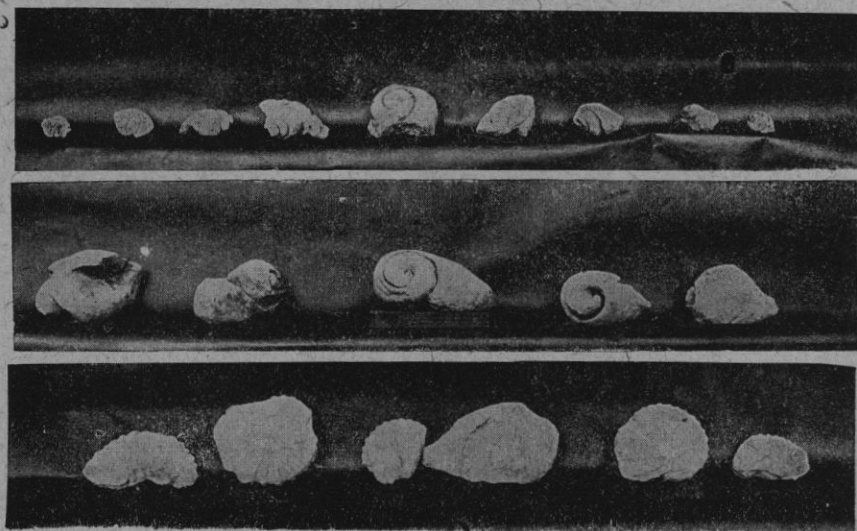
A VII. terem részletei: kőzet és ásványgyűjtemény és megkövült ősi csigák.
